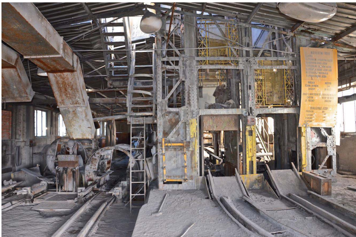
JOM – horní náraží s kruhovými výklopníky.
