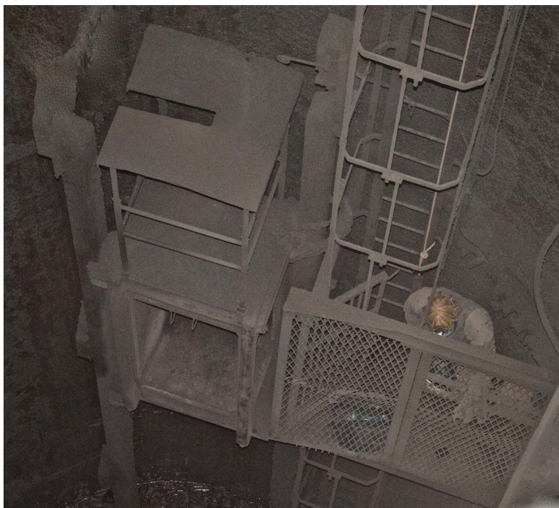
NJJ – stvol jámy několik metrů nad vodou v hloubce cca 15 m. Vlevo pomocná klec pro mužstvo, vpravo lezné oddělení.
